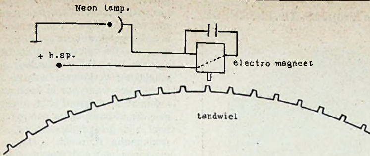
Fig. 1. Baird's automatische synchronisator.
