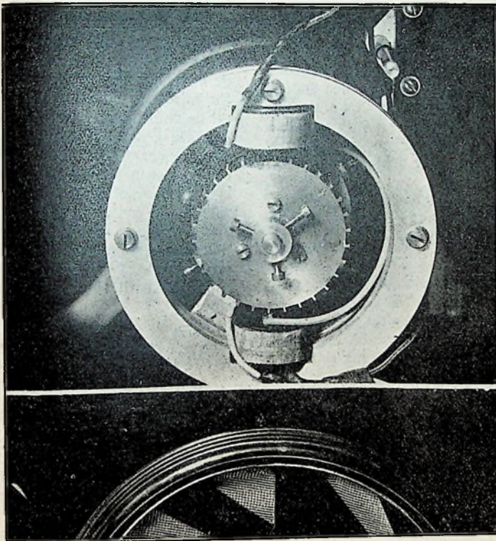
Fig. 2. Baird's automatische Synchronisator.
