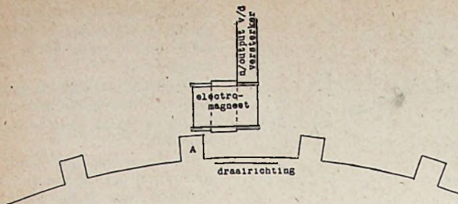
Fig. 4. Dit is de toestand, wanneer de ontvangmotor niet synchroon loopt. De wikkelingen van den electromagneet krijgen thans de stroomvariaties van het beeld en oefenen een remmende werking uit op tandje „A”.
